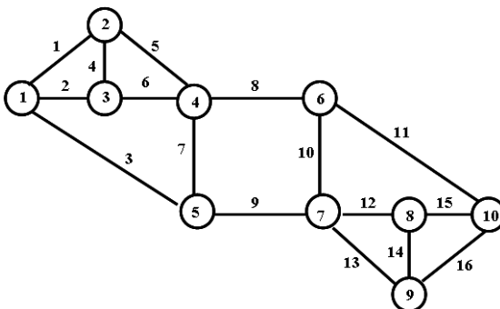
Рис. 8. Граф G_4
