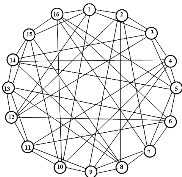
Рис. 5. Сильно регулярный граф G_1 (lattice graph) с параметрами \text{srg}(16,6,2,2)
