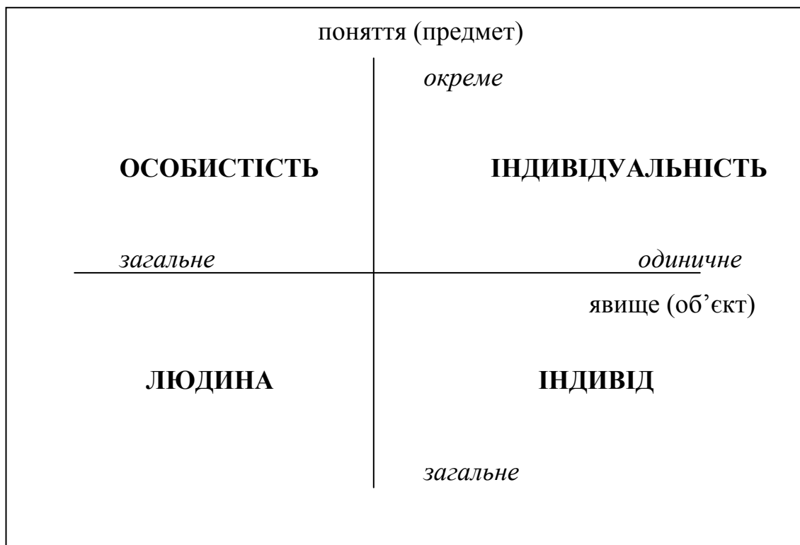
Рис.1. Суб'єкт активності.
