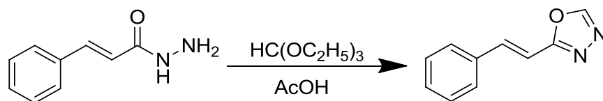
Рис. 12. Синтез 5-незаміщених-2-стирил-1,3,4-оксадіазолів
