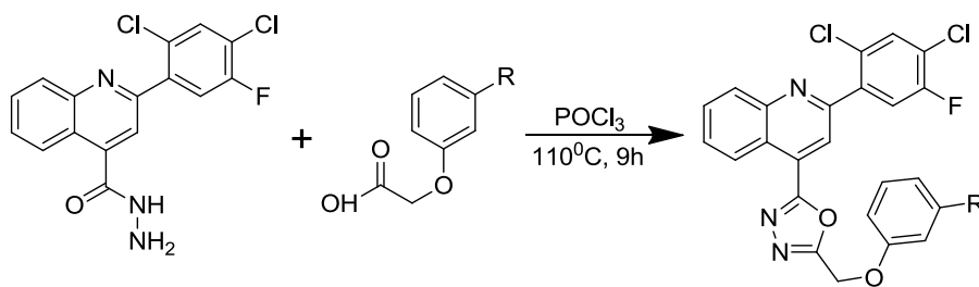
Рис. 8. Синтез 4-([5-(1-метилоксиарил)]-1,3,4-оксадіазол-2-іл)хінолінів
