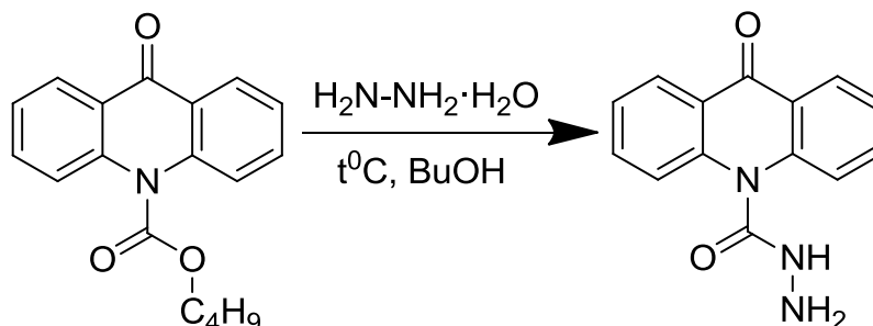
Рис. 4. Синтез гідрозиду акридоноцтової кислоти з іншого естеру
