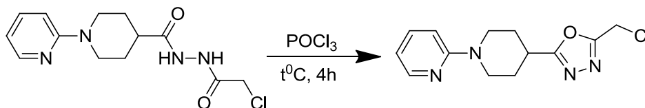
Рис. 6. Синтез 2-(хлорметил)-5-(1-(піридин-2-іл)піперидин-4-іл)-1,3,4-оксадіазолу
