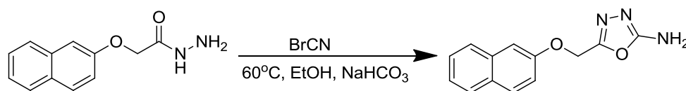
Рис. 14. Синтез 2-аміно-5-(2-нафтілоксиметил)-1,3,4-оксадіазолу
