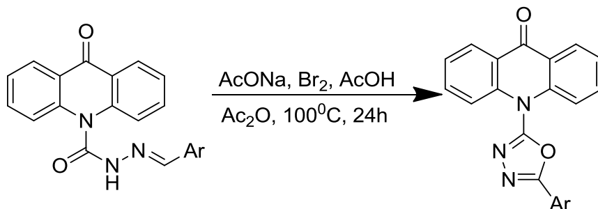
Рис. 5. Синтез 4-(5-заміщені-1,3,4-оксадіазол-іл)акридонів
