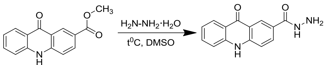
Рис. 2. Синтез гідрозиду 2-карбоксиакридону
