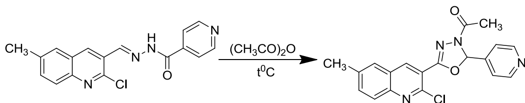
Рис. 10. Синтез 1-(5-(2-хлор-6-метилхінолін-3-іл)-2-(піридин-4-іл)-1,3,4-оксадіазол-3(2H)-іл)метанону
