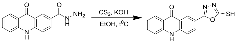
Рис. 11. Синтез 2-(5-меркапто-1,3,4-оксадіазол-2-іл)акридин-9(10H)-ону
